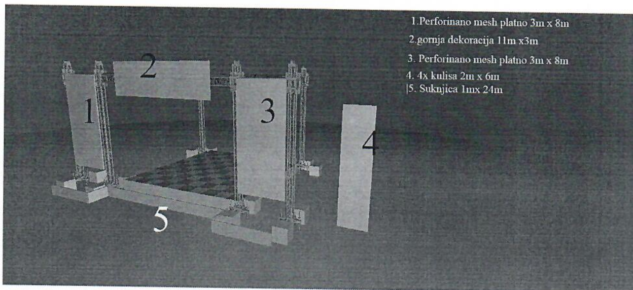
Макет сцены.
